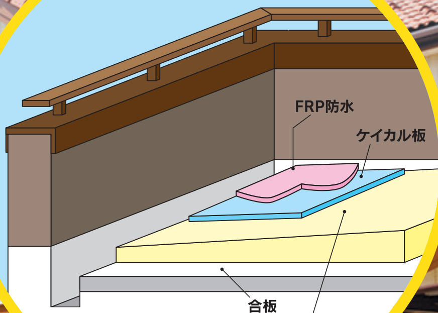
パイナルスロープ施工例
